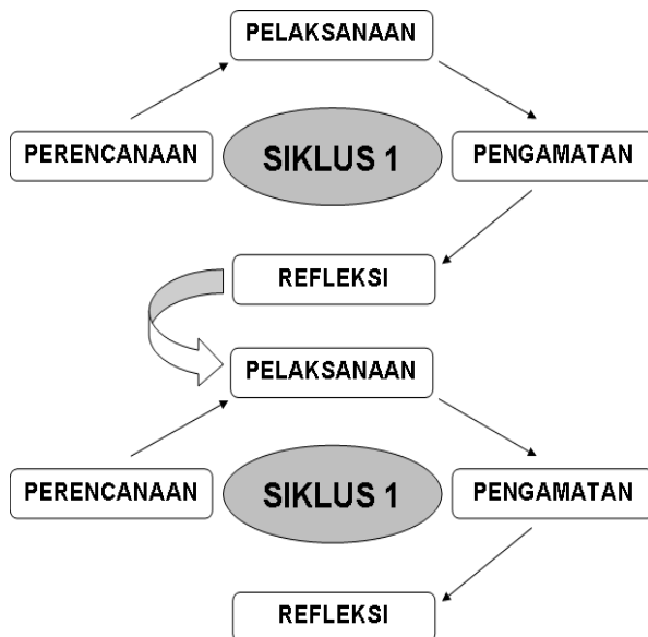
Gambar 1. Siklus Penelitian
